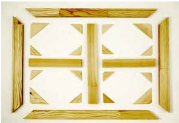
Zusammenbau eines 19 mm Rahmens mit Stütz Kreuz
